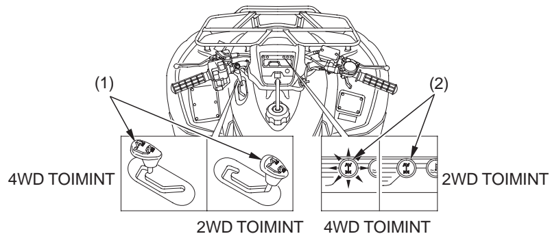
(1) 2WD/4WD valintavipu
