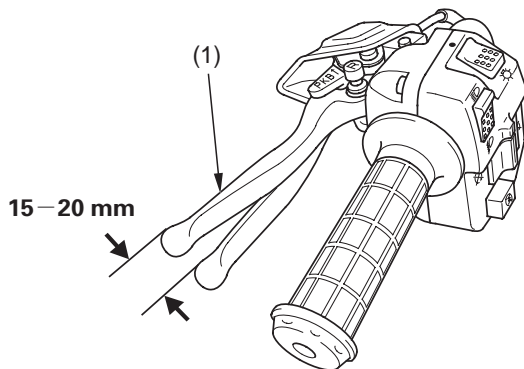
(1) takajarruvipu/pysäköintijarruvipu
