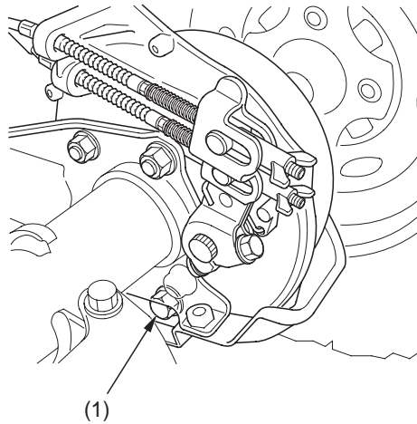
(1) takajarrun tyhjennyspultti
