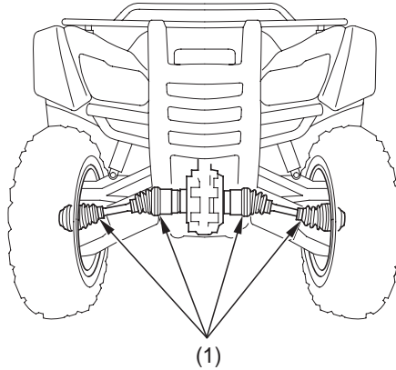
(1) vetoakselin suojakumit
