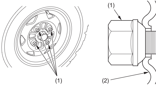
(1) pyörän mutterit
