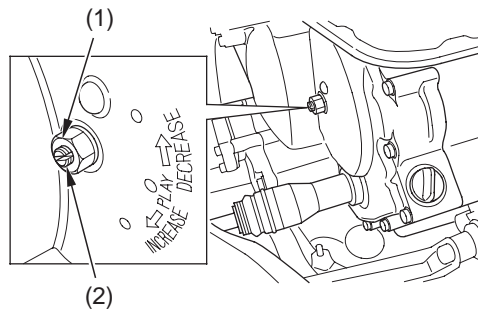
(1) lukkomutteri
